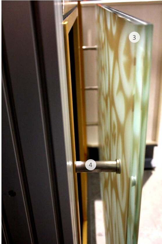
Brüstungsscheibe mit Glashalter Parapet pane with glass holder
